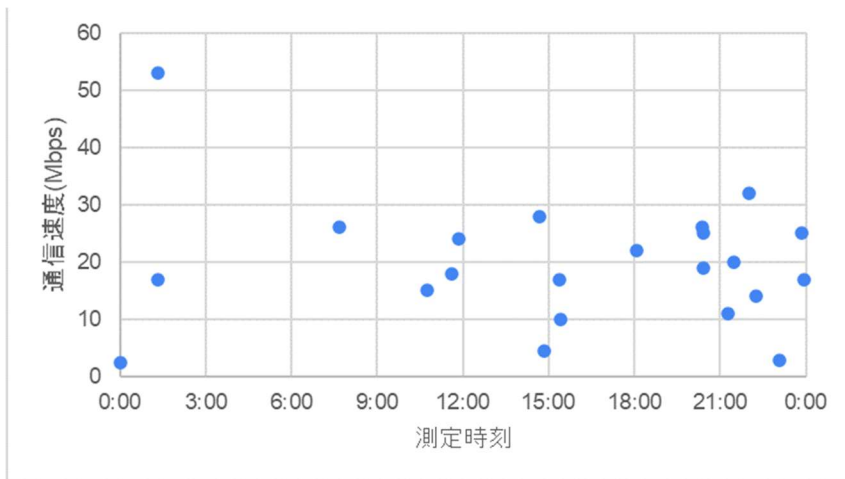
図1 平砂宿舎における各時刻の無線 LAN の通信速度
